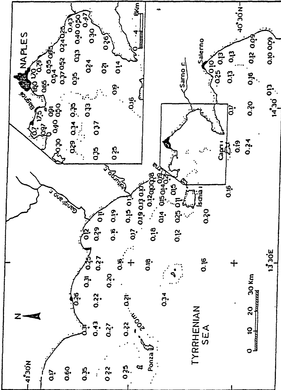
Figure 8. Concentrations de mercure (mg kg -1 de poids sec) à une profondeur de 0 à 3 cm de sédiments du golfe de Naples (Baldi et al., 1983).
