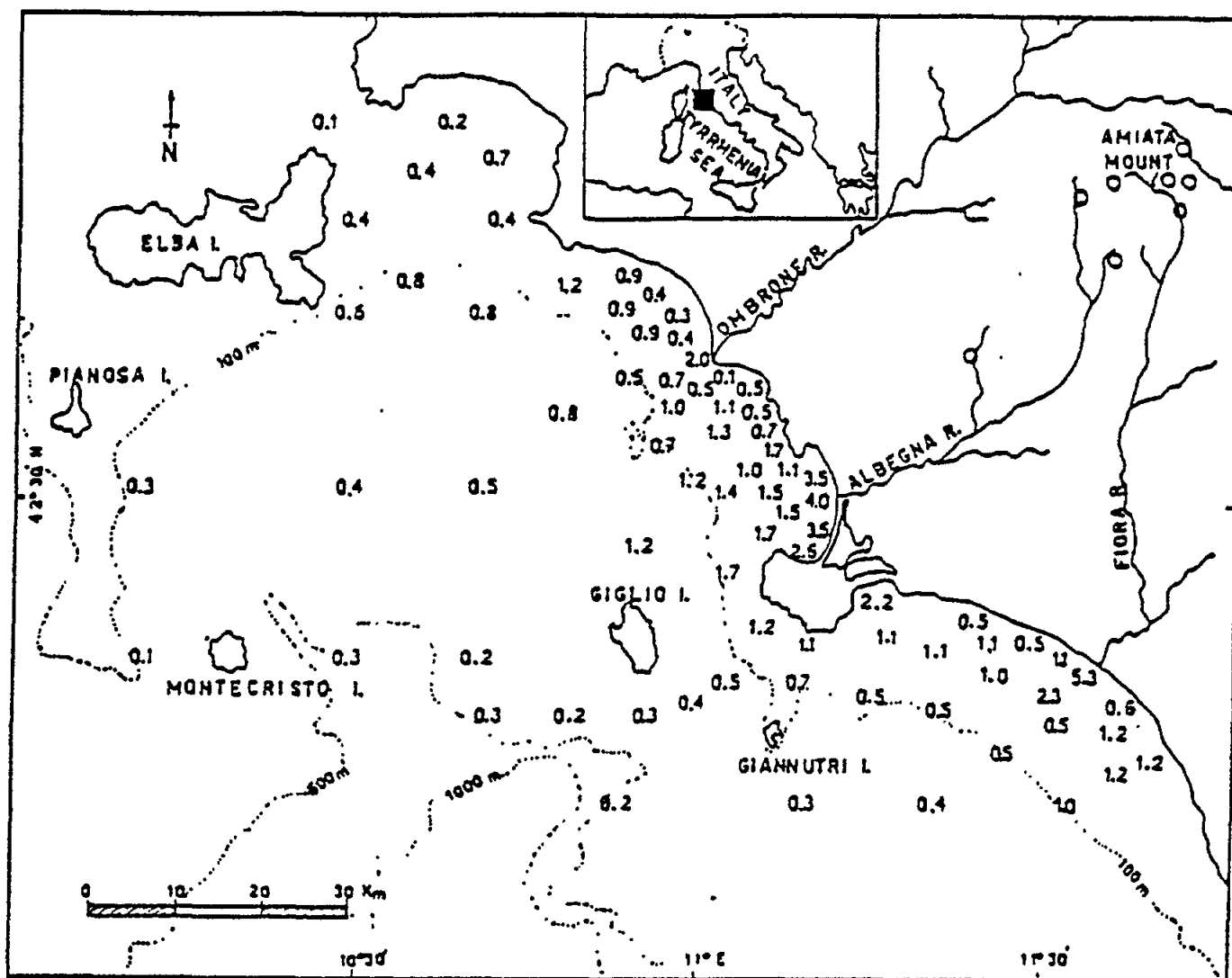
Figure 29. Répartition du mercure ( \text{mg Hg-T Kg}^{-1} de poids sec) dans des sédiments superficiels de la côte ouest de l'Italie, de l'île d'Elbe jusqu'au Fiora (Baldi et Bargagli, 1982). Noter les sites de mines de cinabre (o).
