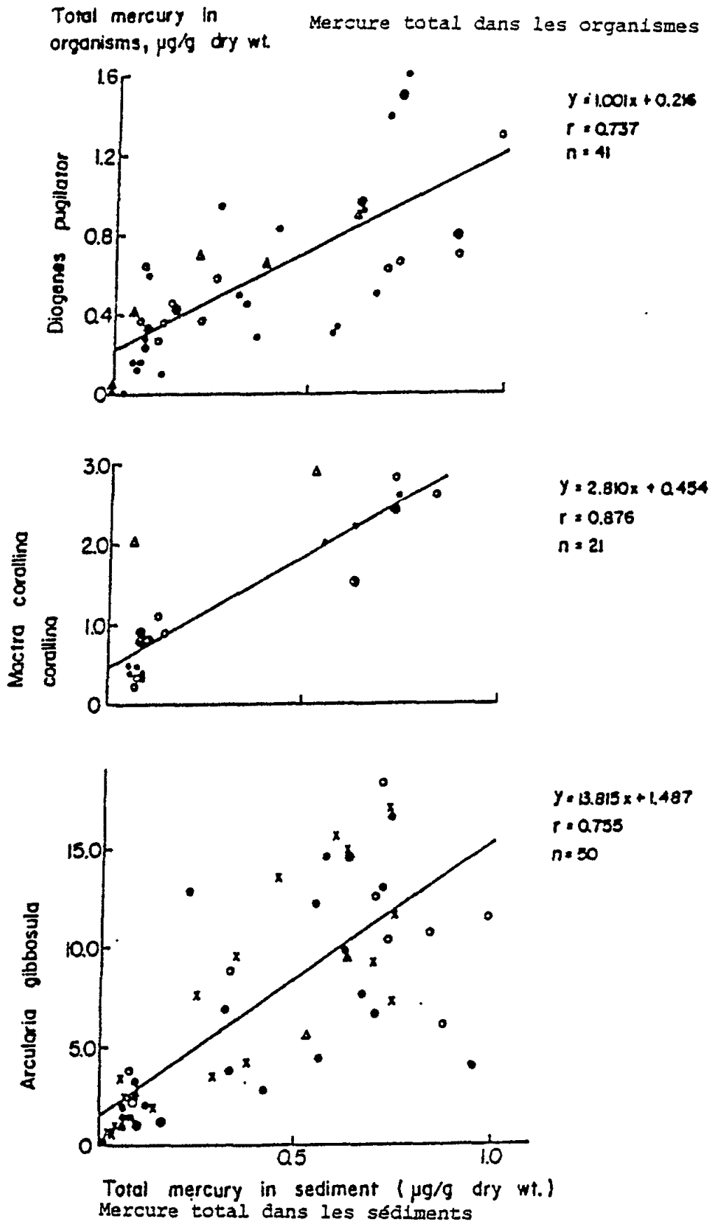
Figure 43. Relation entre les concentrations de mercure dans trois organismes benthiques et des sédiments superficiels du littoral d'Israël (Hornung, 1986). Remarque: chaque point correspond aux teneurs en Hg d'organismes et sédiments échantillonnés à la même date. Symboles: \Delta = juillet 1980 O = juillet 1981 \bullet = sept. 1981 \ast = mai 1982 x = nov./déc. 1982.
