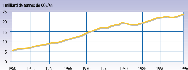
Emissions de dioxyde carbone dans le monde
