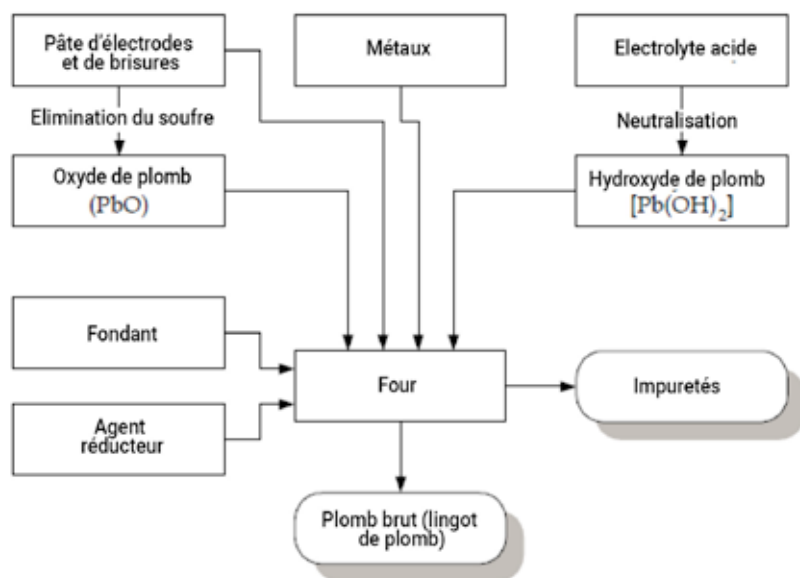
Fig. 30: Diagramme d'un procédé pyrométallurgique de fusion du plomb 1 .
