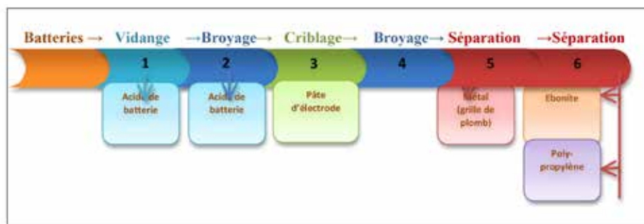
Fig. 17 : Procédé typique de traitement des batteries au plomb usagées 7
