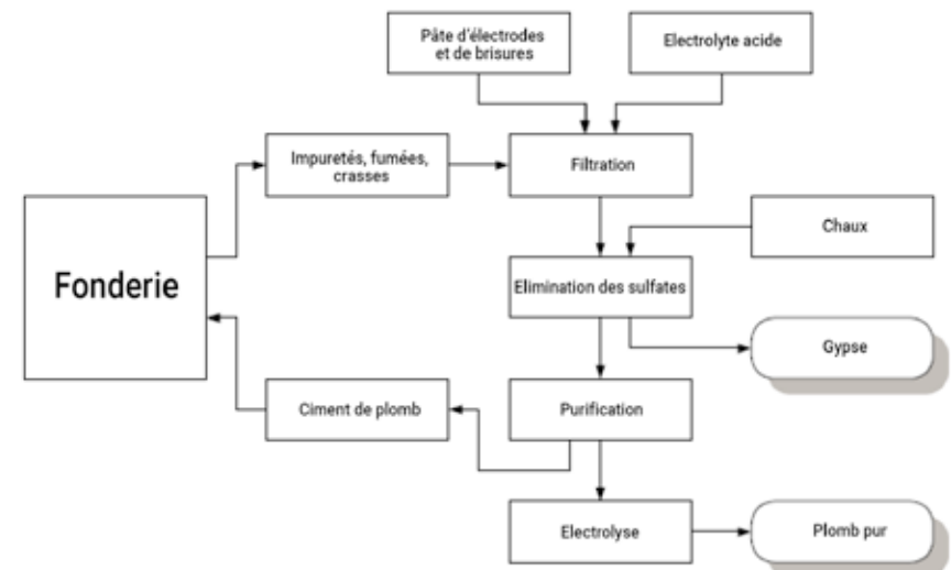
Fig. 28: Diagramme pour l'électrolyse du plomb 1 .
