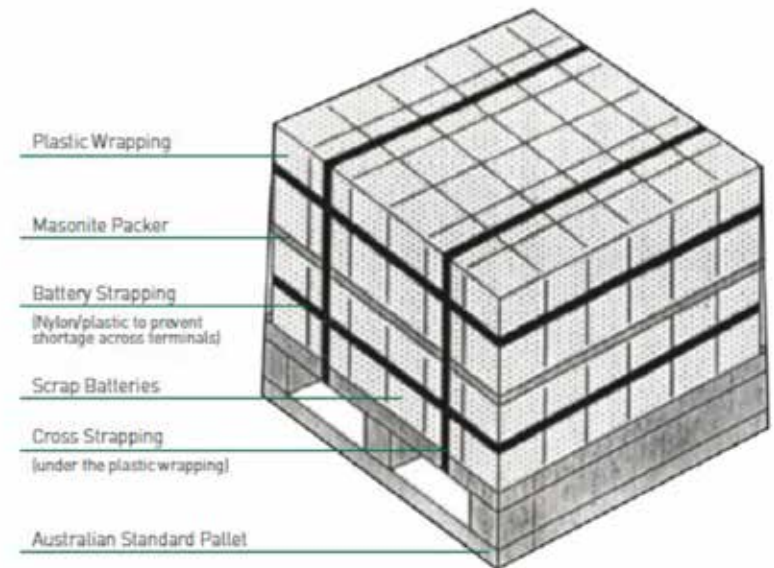
Fig. 14: Exemple de transport correct de batteries au plomb usagées Source: Recyclage responsable des batteries au plomb-acide usagées, Comment maîtriser les risques environnementaux et financiers et de perte de renommée, Initiative australienne pour le recyclage de batteries, ABRI, 26
