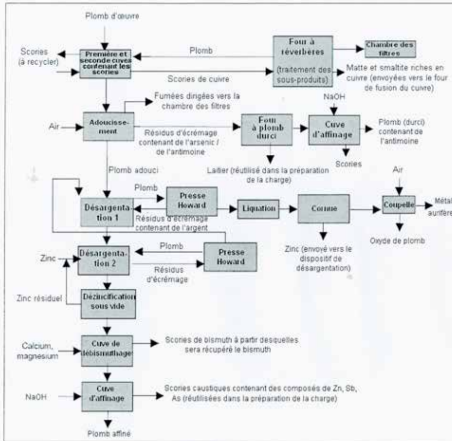
Fig. 31: Diagramme détaillé représentant les procédés d'affinage du plomb 11 .
