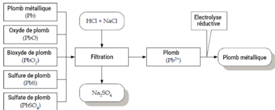
Fig. 29: Procédé électrochimique dans la production de plomb par méthode hydrométallurgique 1 .
