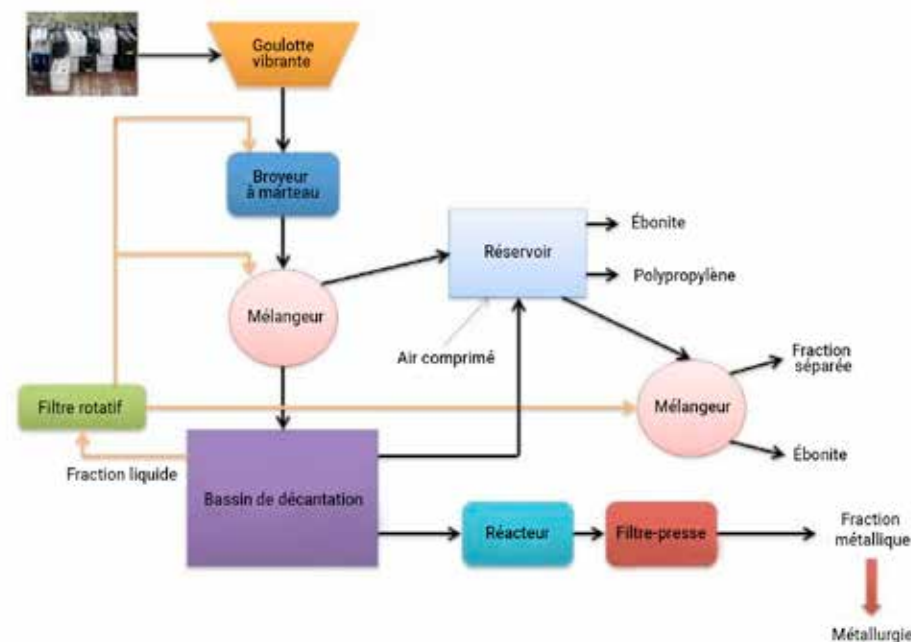
Fig. 21: Exemple de schéma de technologie de traitement humide (Engitec) 16
