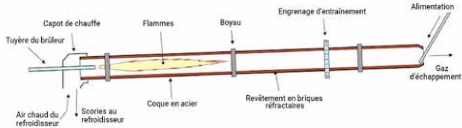
Fig. 25: Exemple de four rotatif 30 .
