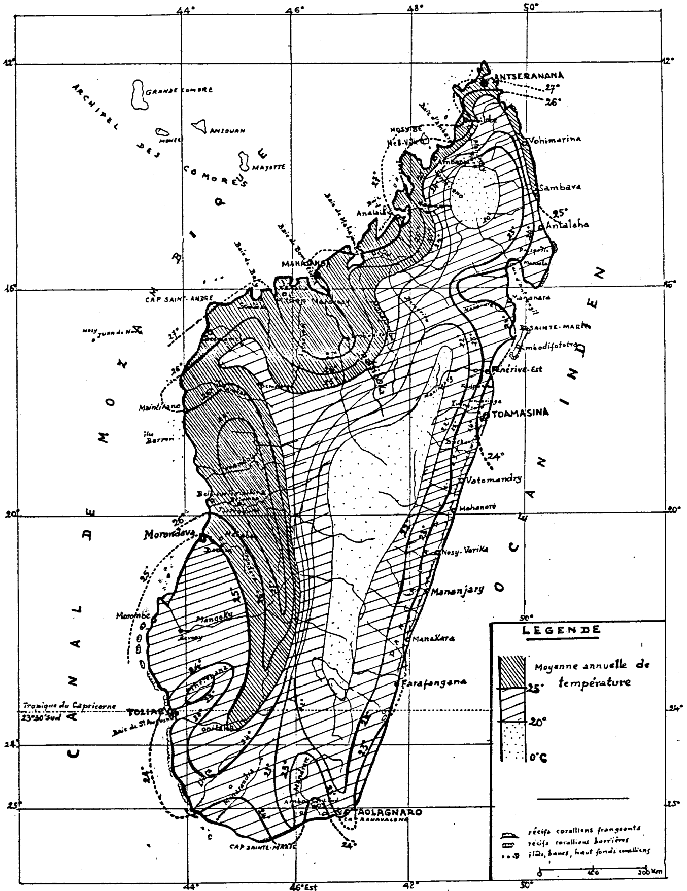
Carte 4: Isothermes annuelles des régions cotières Malgaches
