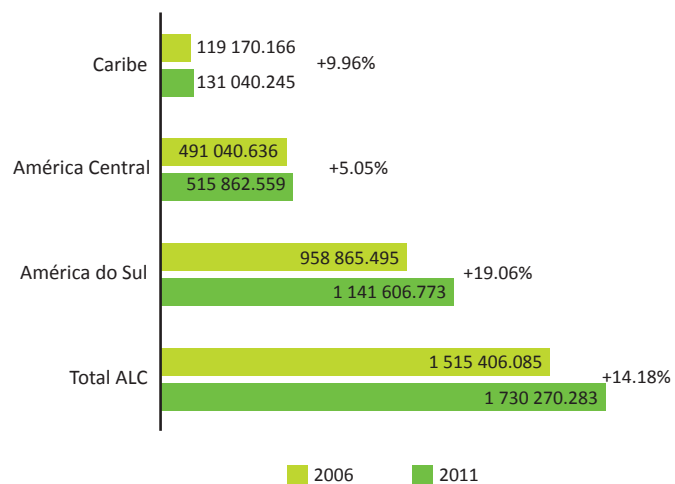
Figura 2.1.9: Total de emissões de dióxido de carbono em 2006 e 2011 (kg por ton. por ano) nas sub-regiões da ALC.
