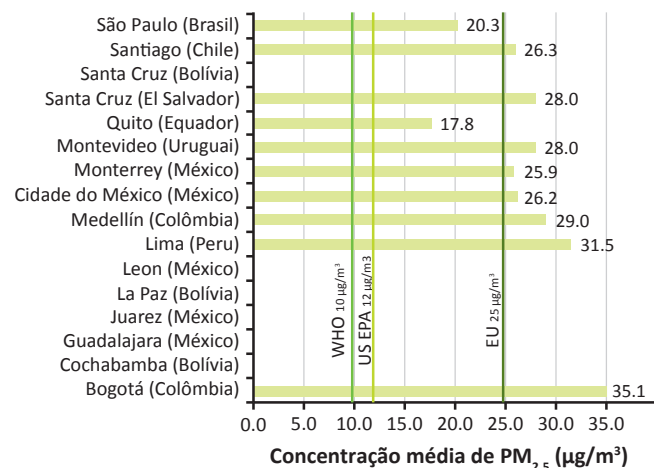
Figura 2.1.3: Média anual de concentrações de PM_{2.5} e PM_{10} ( \mu g m^{-3} ) em cidades selecionadas na América Latina e no Caribe (2011). As linhas verticais representam os padrões de qualidade para PM de OMS, US-EPA e UE definidos como a média anual de quantidade máxima de particulados que podem estar presentes no ar exterior sem ameaçar a saúde pública.
