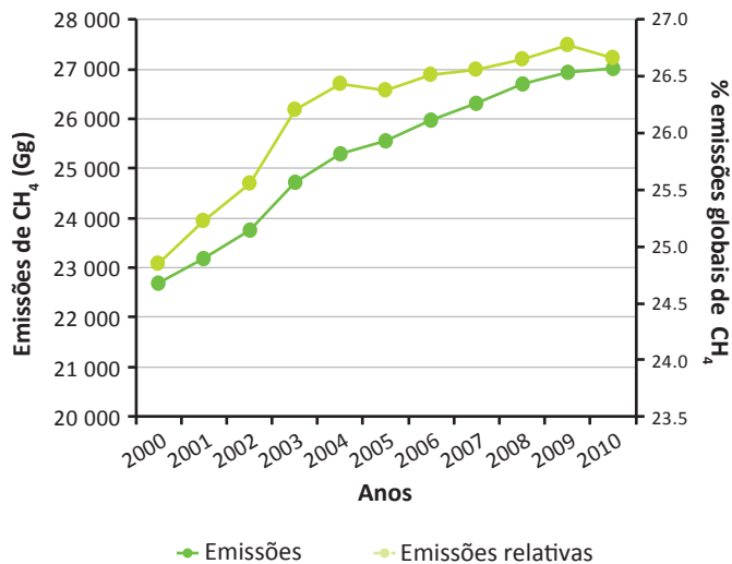
Figura 2.1.8: Emissões de metano ( CH_4 ) da ALC provenientes da fermentação entérica do gado (eixo esquerdo) e sua participação relativa nas emissões globais totais de metano da mesma fonte (eixo direito).
