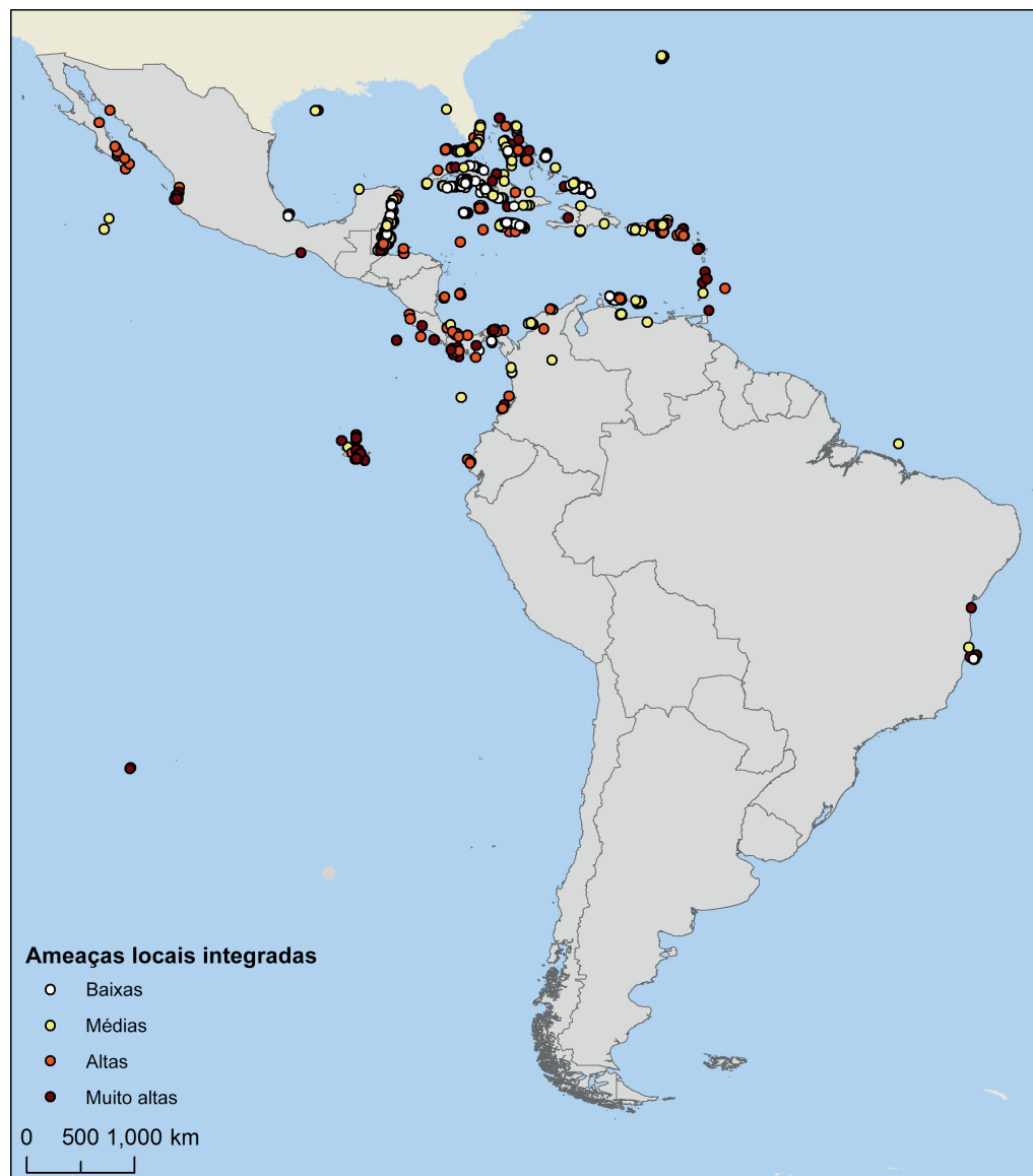
Figura 2.5.7: Recifes de coral classificados por ameaças locais integradas (2014).
