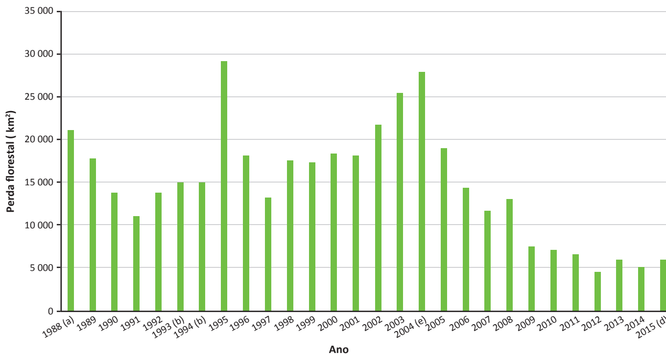
Figura 2.5.5: Taxas de desmatamento na Amazônia brasileira, 1988-2015
