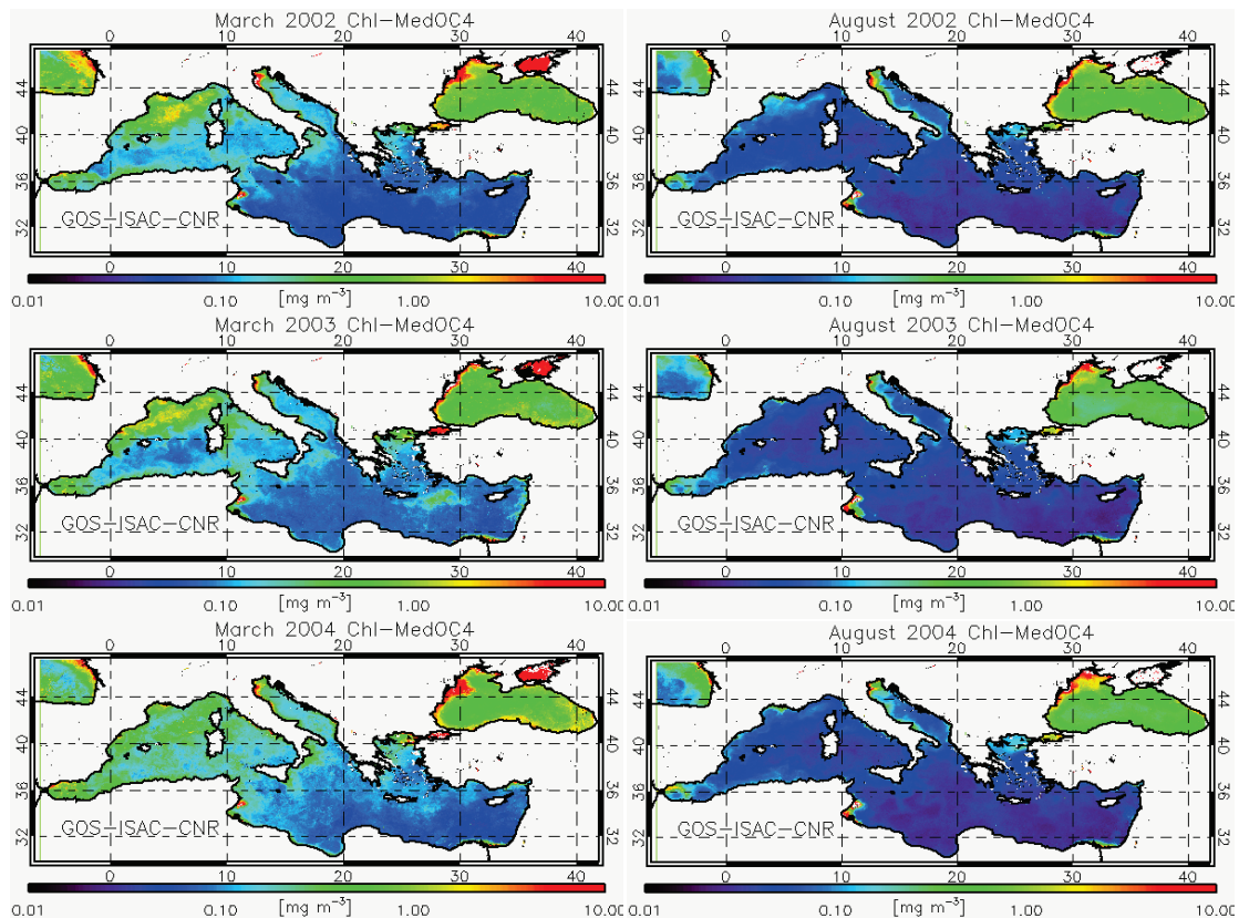
Figure 13 Concentrations de chlorophylle en mer Méditerranée, 2002-2004
