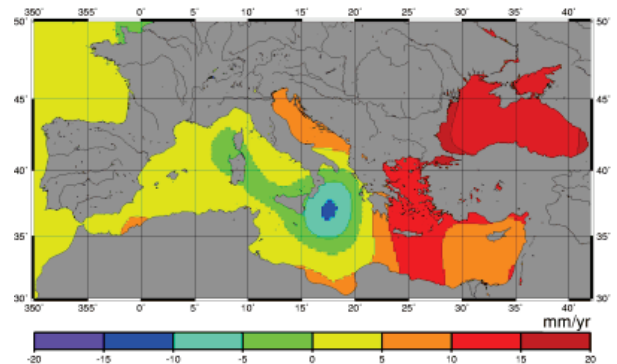
Figure 6 Variations du niveau de la mer observée entre 1999 et 2006 par le projet TOPEX/Poséidon (mm/année)
