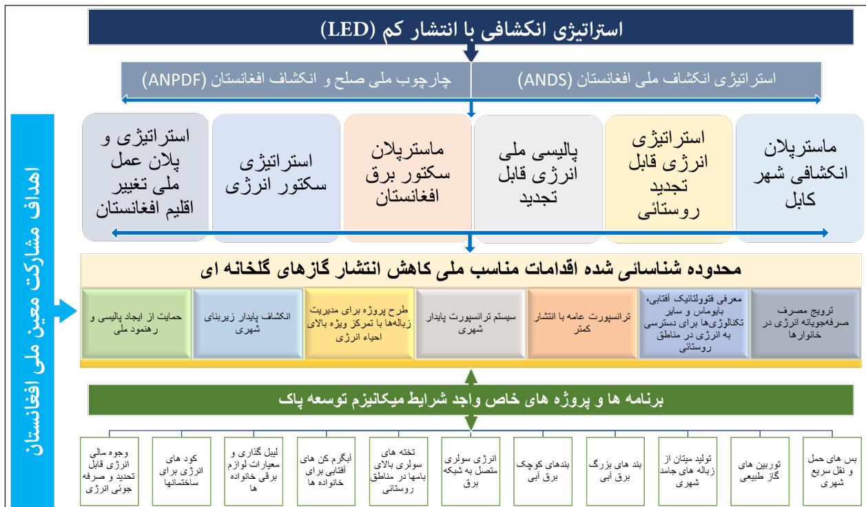
شکل ۵۸: سلسله منطقی تعیین فعالیت‌های کاهش انتشار گازهای گلخانه که از استراتژی‌های انکشافی با انتشار کم آغاز میگردد
