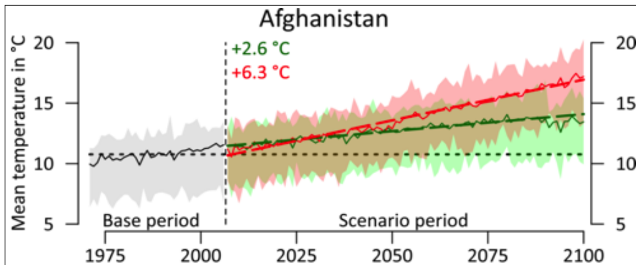
شکل ۱۰: پیش‌بینی های اوسط بارندگی سالانه افغانستان بین سال‌های ۱۹۷۵ الی ۲۱۰۰ ۲۹
