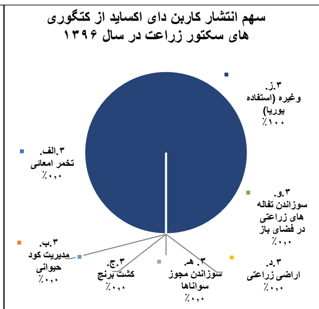
شکل ۴۶: انتشار کاربن دای اکساید از سکتور زراعت در سال ۱۳۹۶
