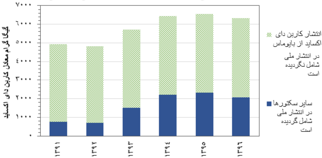
شکل ۳۹: انتشار کاربن دای اکساید ناشی از احتراق بایوماس برای تولید انرژی بین سالهای ۱۳۹۱ الی ۱۳۹۶
