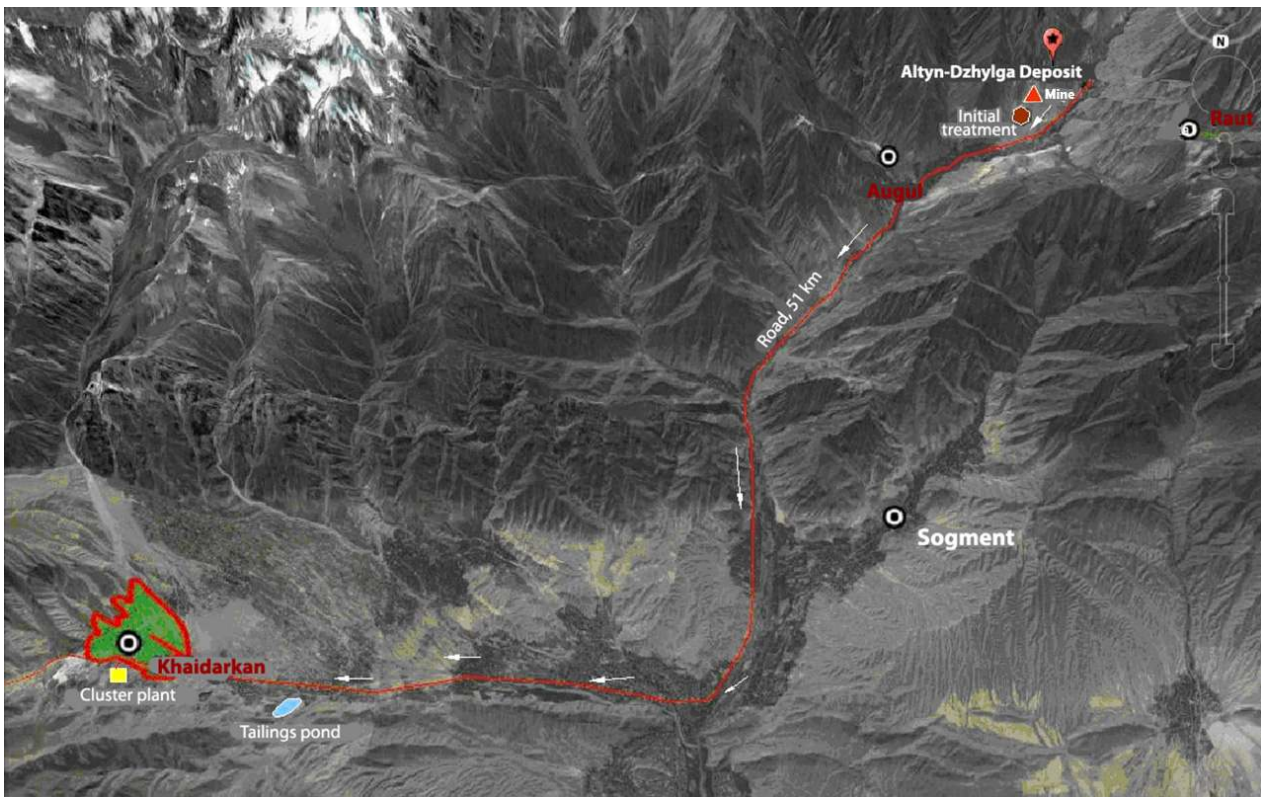
Fig. 1.1 Location of Alтын-Dzhyлга deposit
