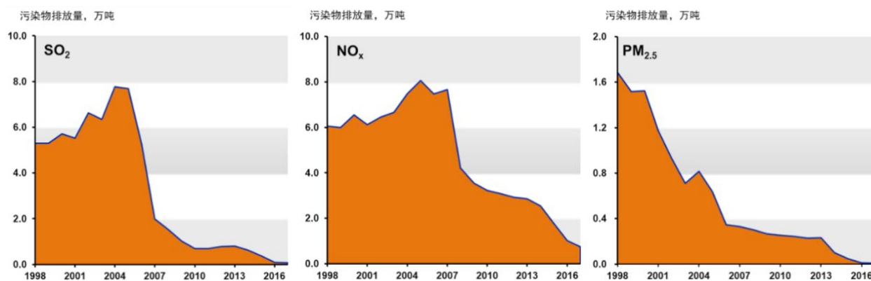
图 5 北京市电厂的污染控制成效，1998-2017 年
