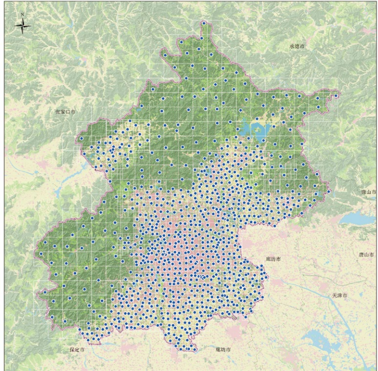
图 3 北京市高密度 PM_{2.5} 传感器监测网络
