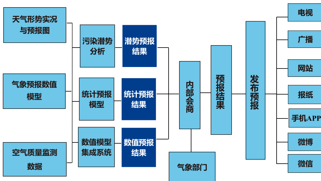
图 3.6 北京环境空气质量预报技术体系和业务组成
