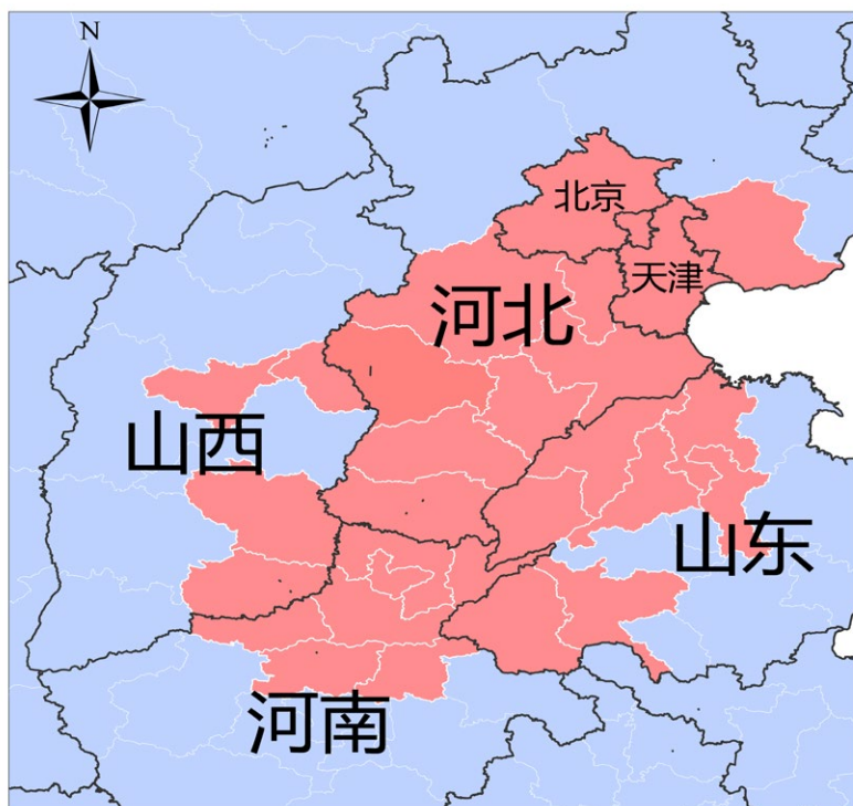
图 5.1 京津冀及周边地区“2+26”城市(图中红色区域)分布图
