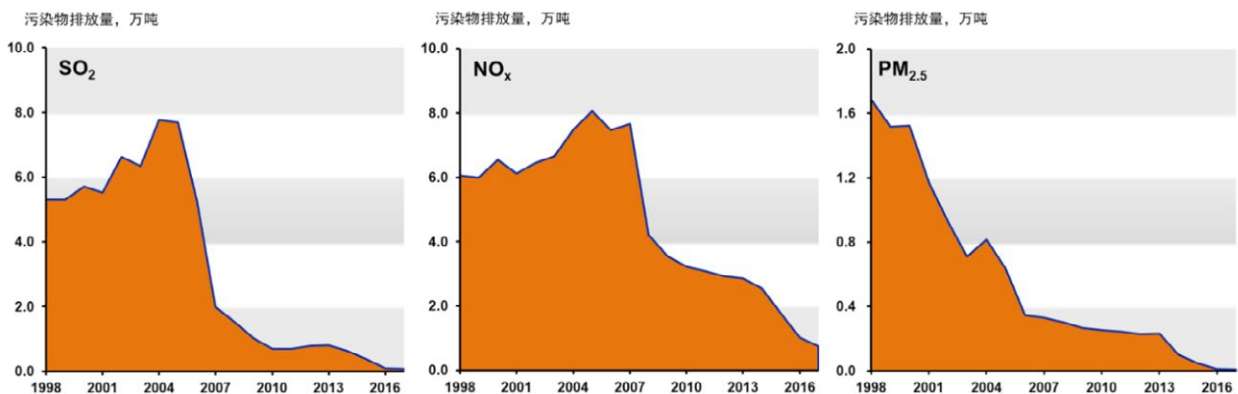
图 4.5 北京市 1998-2017 年间电厂主要大气污染物排放情况
