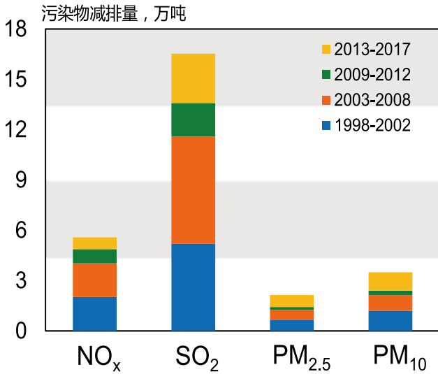
图 4.6 北京市 1998-2017 年间燃煤锅炉改造污染物减排量
