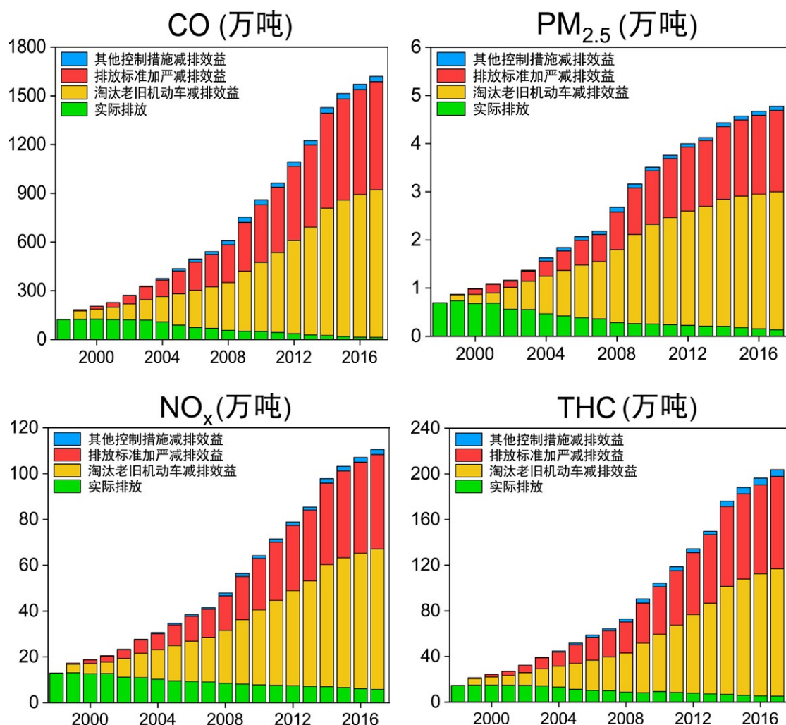
图 4.7 北京市 1998-2017 年间移动源实际排放及管控措施减排效益
