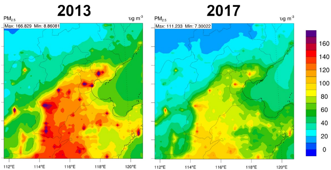
图 6.5 北京及周边地区 PM 2.5 年均浓度的空间分布 (2013, 2017)
