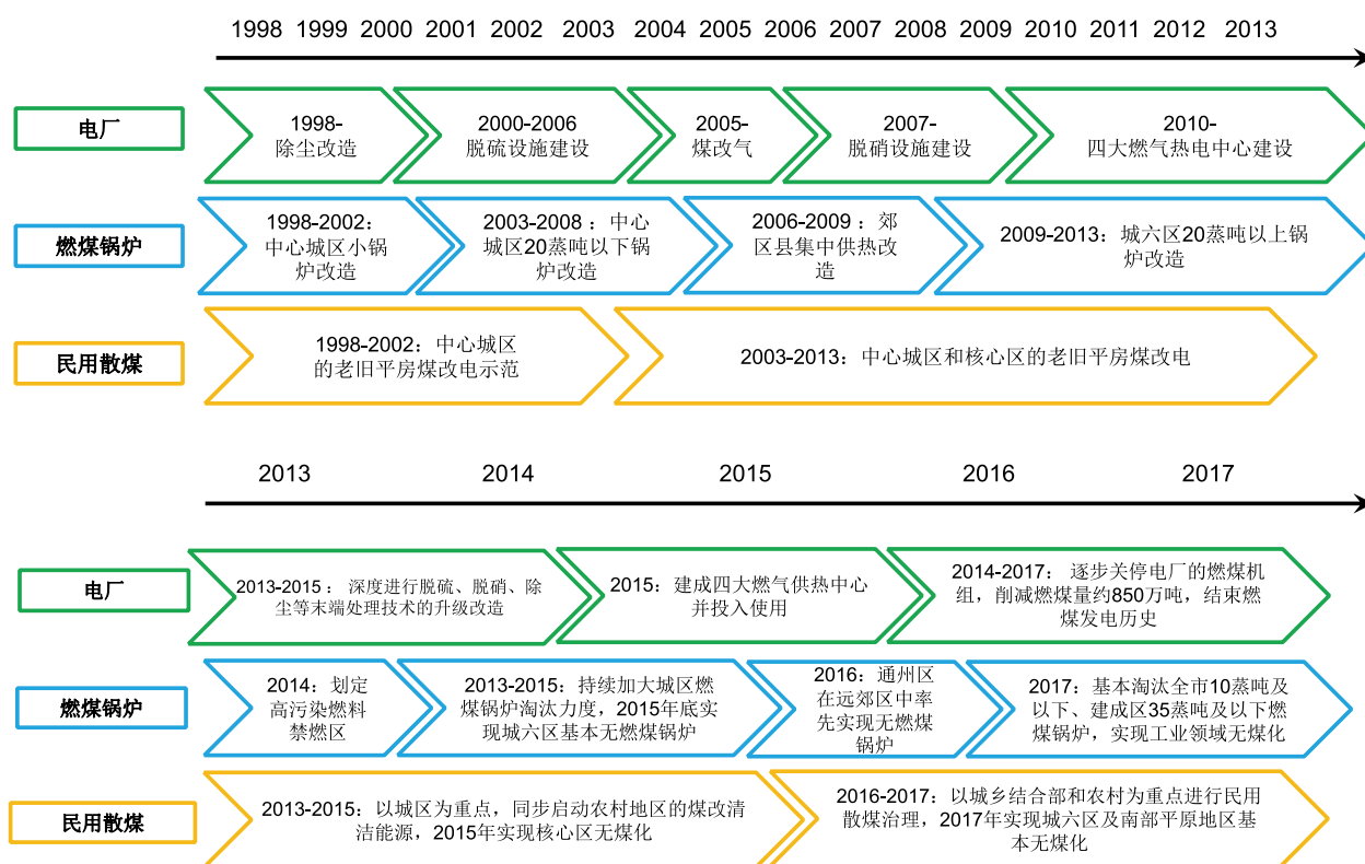
图 4 1998-2017 年期间北京市燃煤源污染控制过程及措施
