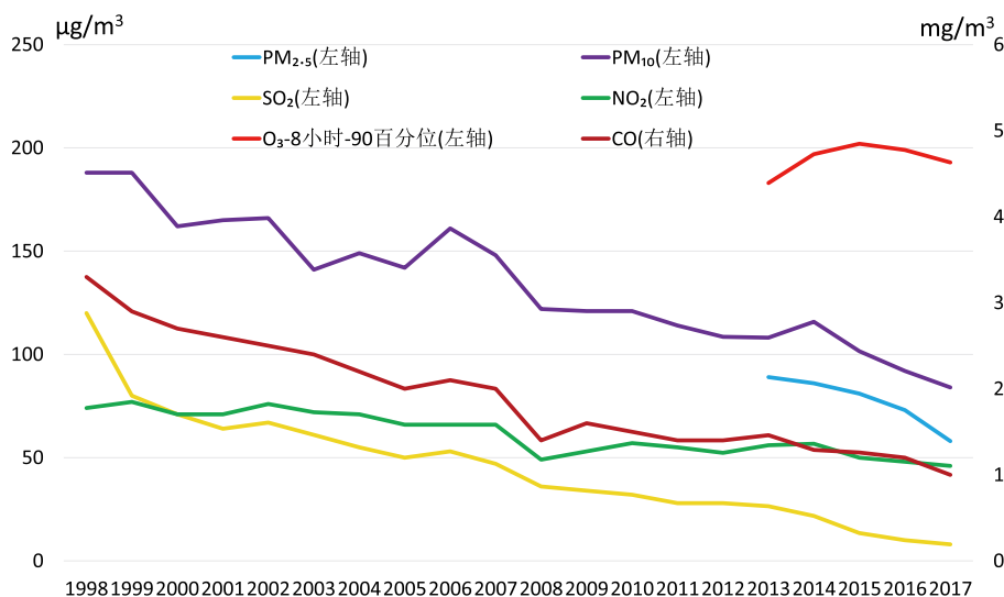
图 1 北京市主要空气污染物年均浓度变化，1998-2017 年
