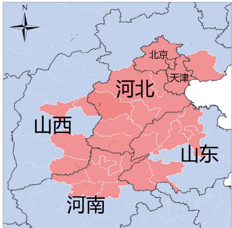
图 10 京津冀及周边地区“2+26”大气污染传输通道城市(图中红色部分)分布图
