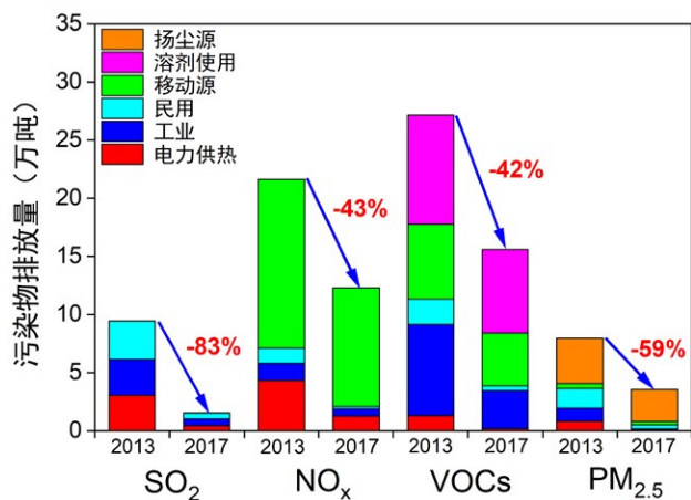
图 6.2 2013-2017 年间北京市主要污染物的排放变化情况
