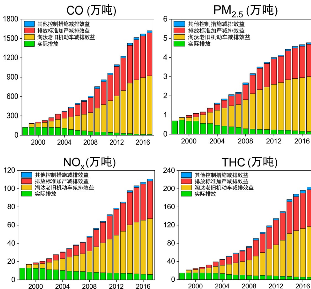
图 8 北京市机动车污染物排放控制措施效益
