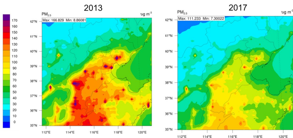
图 11 2013-2017 年北京市及周边地区的 PM 2.5 污染显著改善
