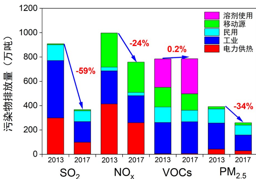
图 5.4 2013-2017 年北京市周边（含天津、河北、河南、山东、山西、内蒙古）主要大气污染物排放变化特征
