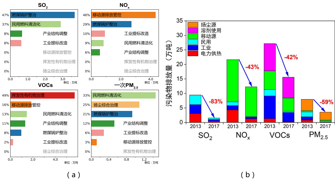
图9 北京 2013-2017 年间减排措施的减排量与相对贡献 (a) , 主要污染物的排放变化情况 (b)
