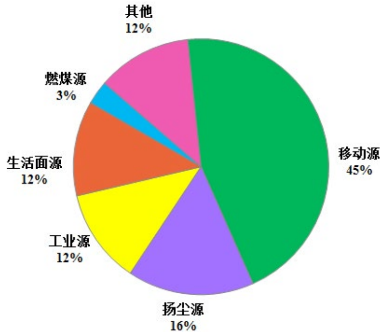
图 2.4 2017 年北京市大气 PM 2.5 来源解析结果—本地来源
