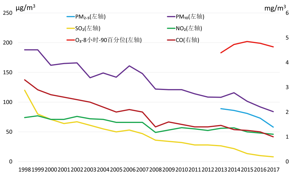
图 2.1 北京市主要大气污染物年均浓度变化趋势，1998-2017
