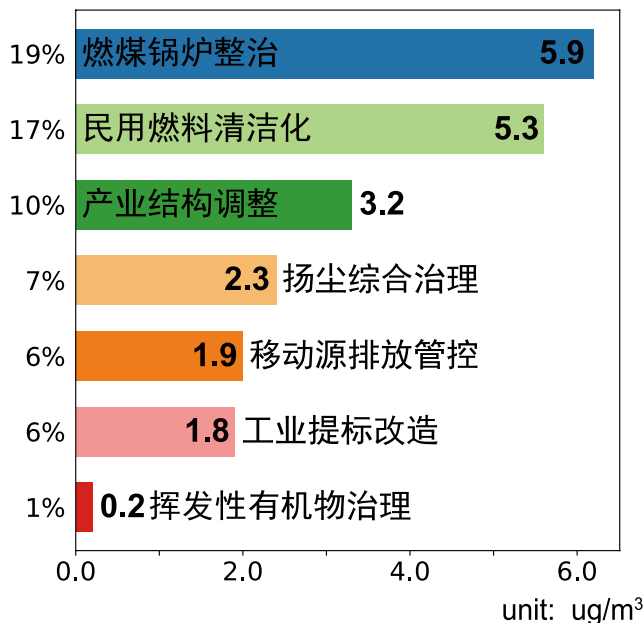
图 6.3 本地减排措施对北京市 2013 至 2017 年 PM 2.5 浓度下降的贡献
