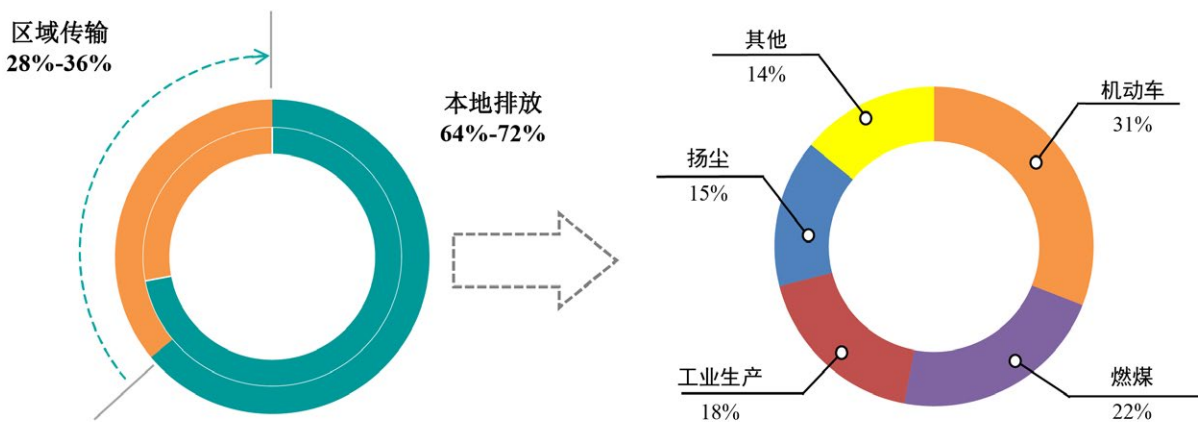
图 2.3 2013 年北京市大气中 PM 2.5 的源解析结果
