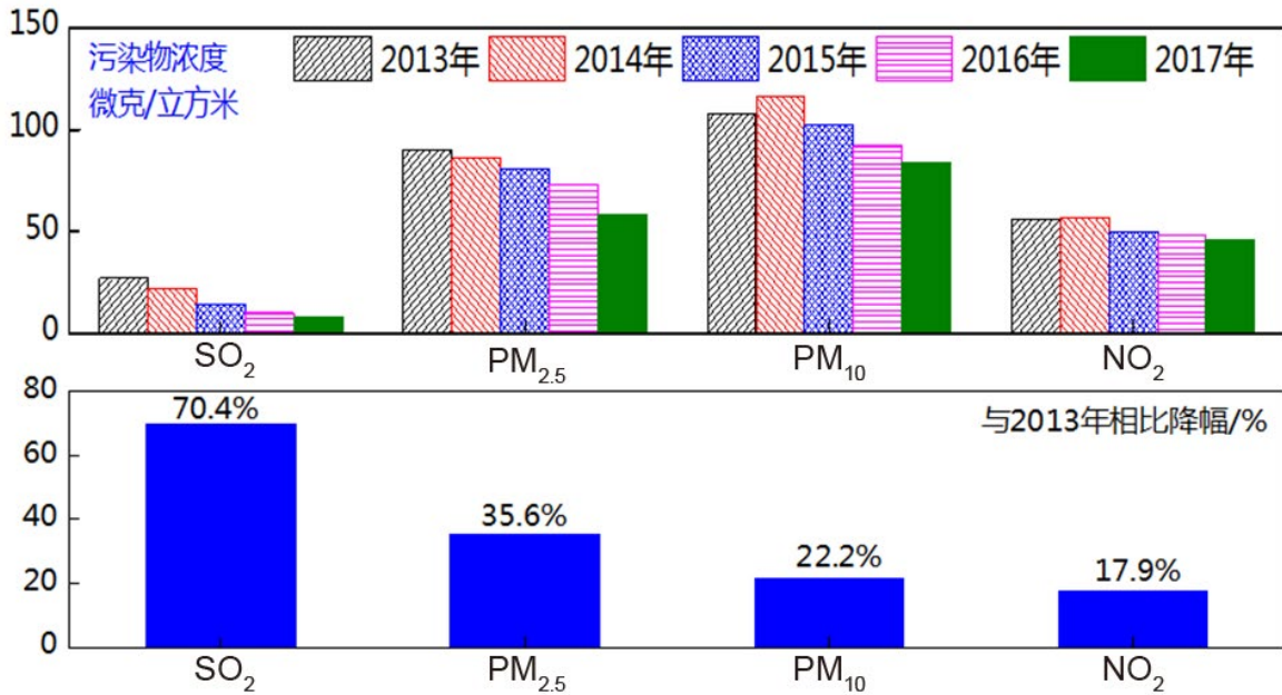
图 2.2 2013-2017 年北京市各项污染物年均浓度及下降幅度
