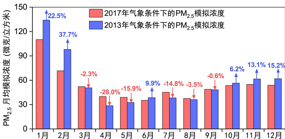
图 6.4 北京市 2017 年排放水平在 2013、2017 年气象条件下的逐月 PM_{2.5} 浓度模拟结果
