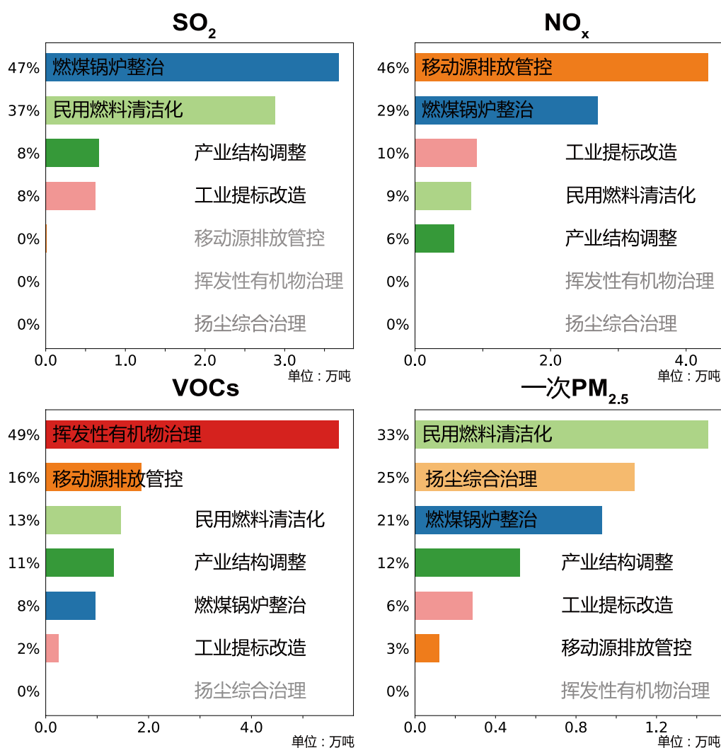
图 6.1 主要措施对 2013-2017 年间北京市主要污染物的减排贡献
