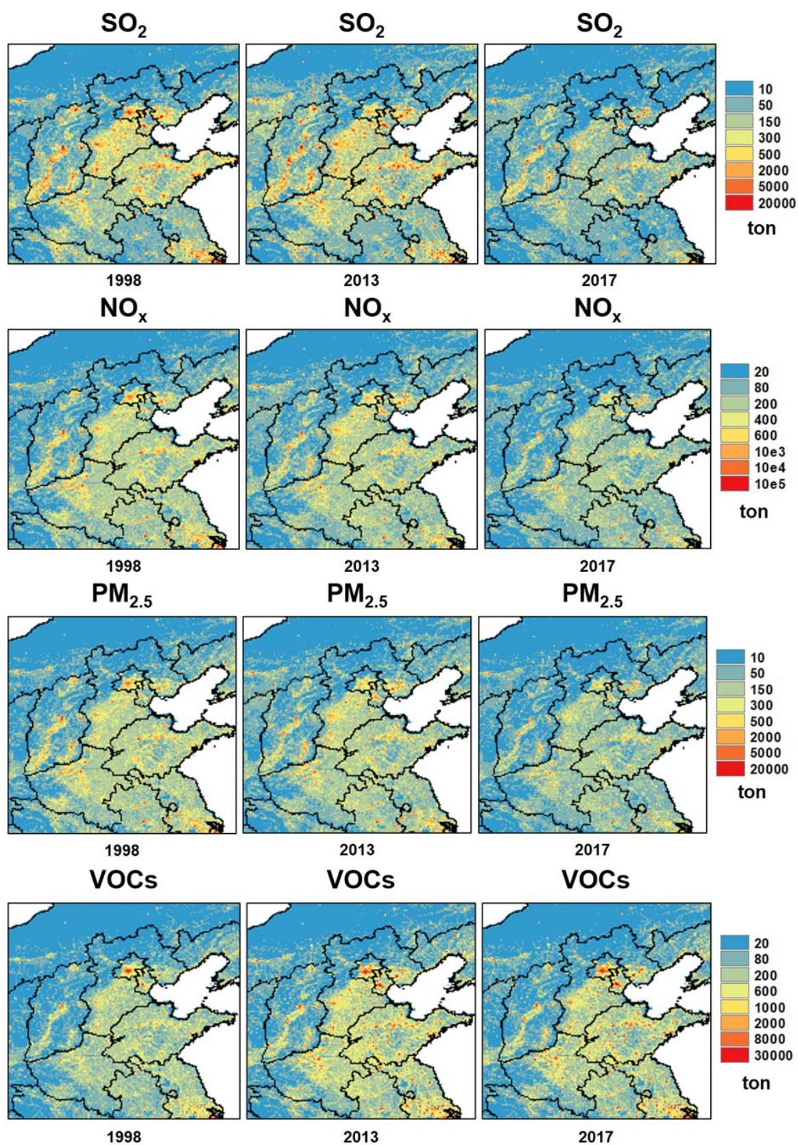
图 5.2 北京市及周边地区 1998、2013 及 2017 年主要污染物排放空间分布
