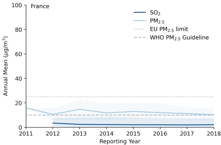
Graphique 8.3-16 : Concentrations moyennes annuelles de SO_2 et de PM_{2,5} en France (les zones ombrées montrent un IC à 95 %)
