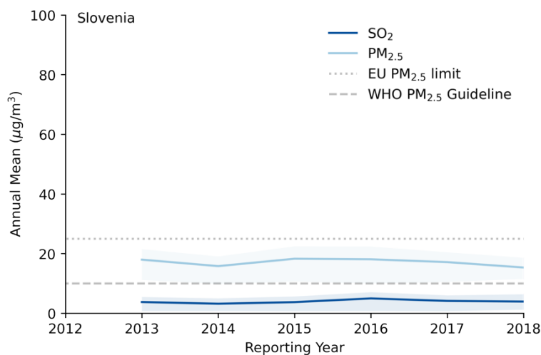
Graphique 8.3-36 : Concentrations moyennes annuelles de SO 2 et de PM 2,5 en Slovénie (les zones ombrées montrent un IC à 95 %)
