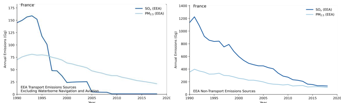
Graphique 8.3-15 : Émissions de SO x et de PM 2,5 dans les transports (à gauche) et hors transports (à droite) en France
