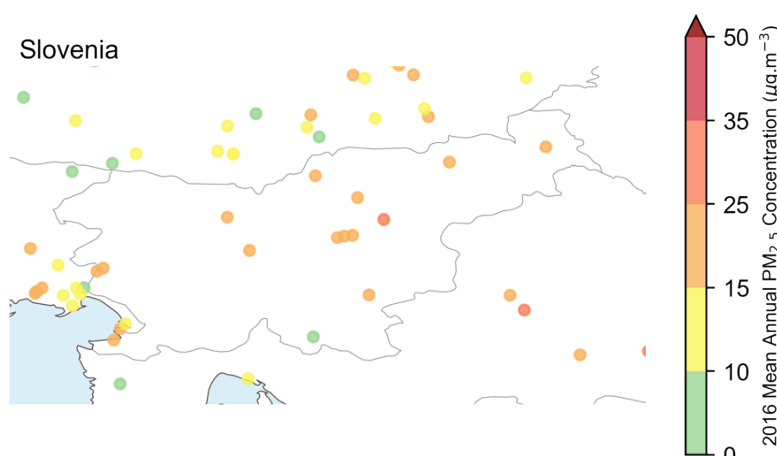
Graphique 8.3-37 : Relevé de l’OMS des concentrations moyennes annuelles de PM 2,5 en Slovénie (2016)
