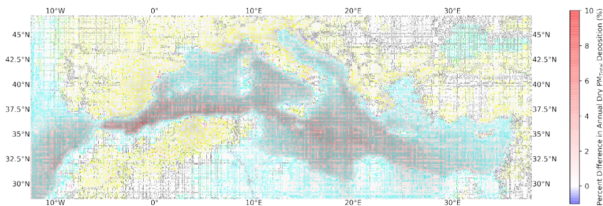
Graphique 5.2-8. Changements en pourcentage des dépôts secs annuels de PM_{Totales} entre MARPOL VI et l'ECA SO_x Med proposée
