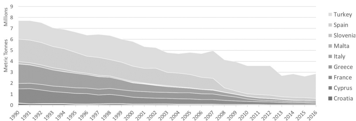
Graphique 1. Évolution des émissions de SO x sur terre pour les États riverains de la mer Méditerranée membres de l'Union européenne ainsi que pour la Turquie
