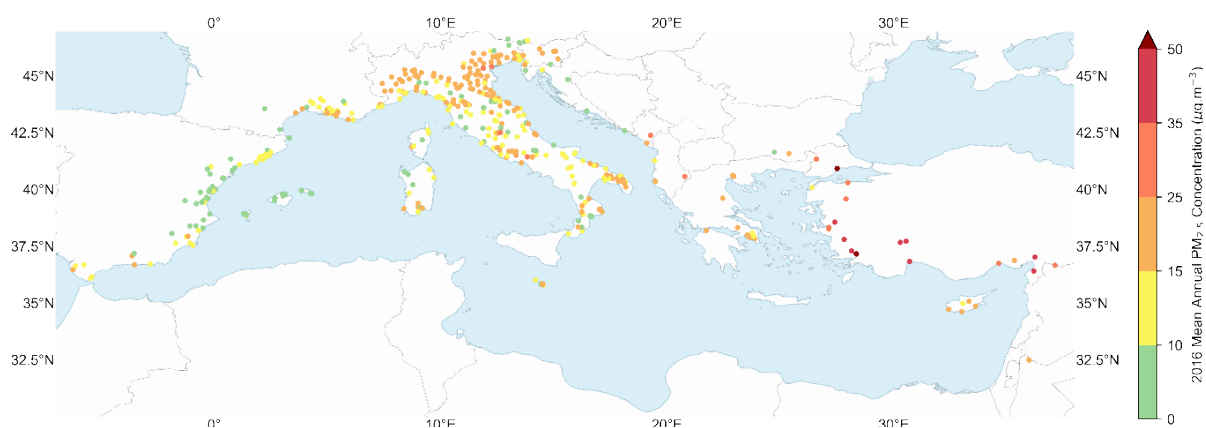
Graphique 8.3-3 : Qualité moyenne annuelle de l'air (PM 2,5 µg/m 3 ) observée aux stations d'observation côtières (à moins de 100 km du littoral)
