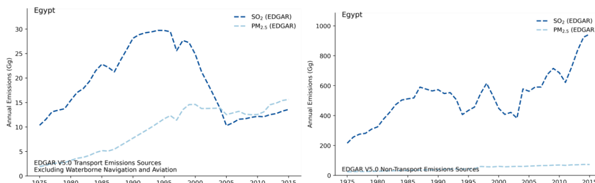
Graphique 8.3-14 : Émissions de SO 2 et de PM 2,5 dans les transports (à gauche) et hors transports (à droite) en Égypte
