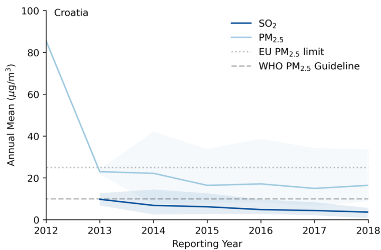
Graphique 8.3-9 : Concentrations annuelles moyennes de \text{SO}_2 et de \text{PM}_{2.5} en Croatie (les zones ombrées montrent une IC à 95 %)
