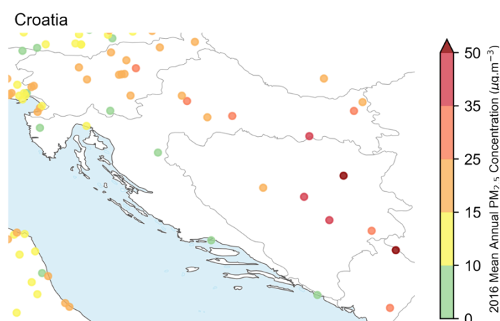
Graphique 8.3-10 : Relevé de l'OMS des concentrations moyennes annuelles de \text{PM}_{2.5} en Croatie (2016)
