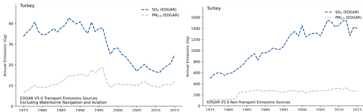
Graphique 8.3-43 : Émissions de SO 2 et de PM 2,5 dans les transports (à gauche) et hors transports (à droite) en Turquie
