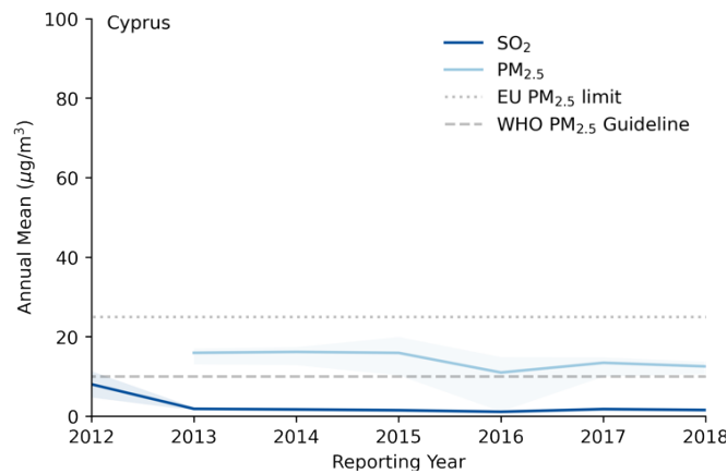
Graphique 8.3-12 : Concentrations moyennes annuelles de SO 2 et de PM 2,5 à Chypre (les zones ombrées montrent un IC à 95 %)
