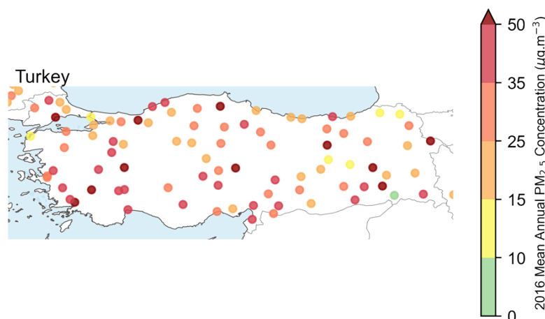
Graphique 8.3-44 : Relevé de l'OMS des concentrations moyennes annuelles de PM 2,5 en Turquie(2016)
