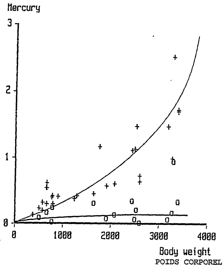
Figure 19. Concentration de mercure ( \text{mg kg}^{-1} ) total (o) et inorganique (+) dans le muscle foncé de Sarda sarda (Capelli et al., 1986).
