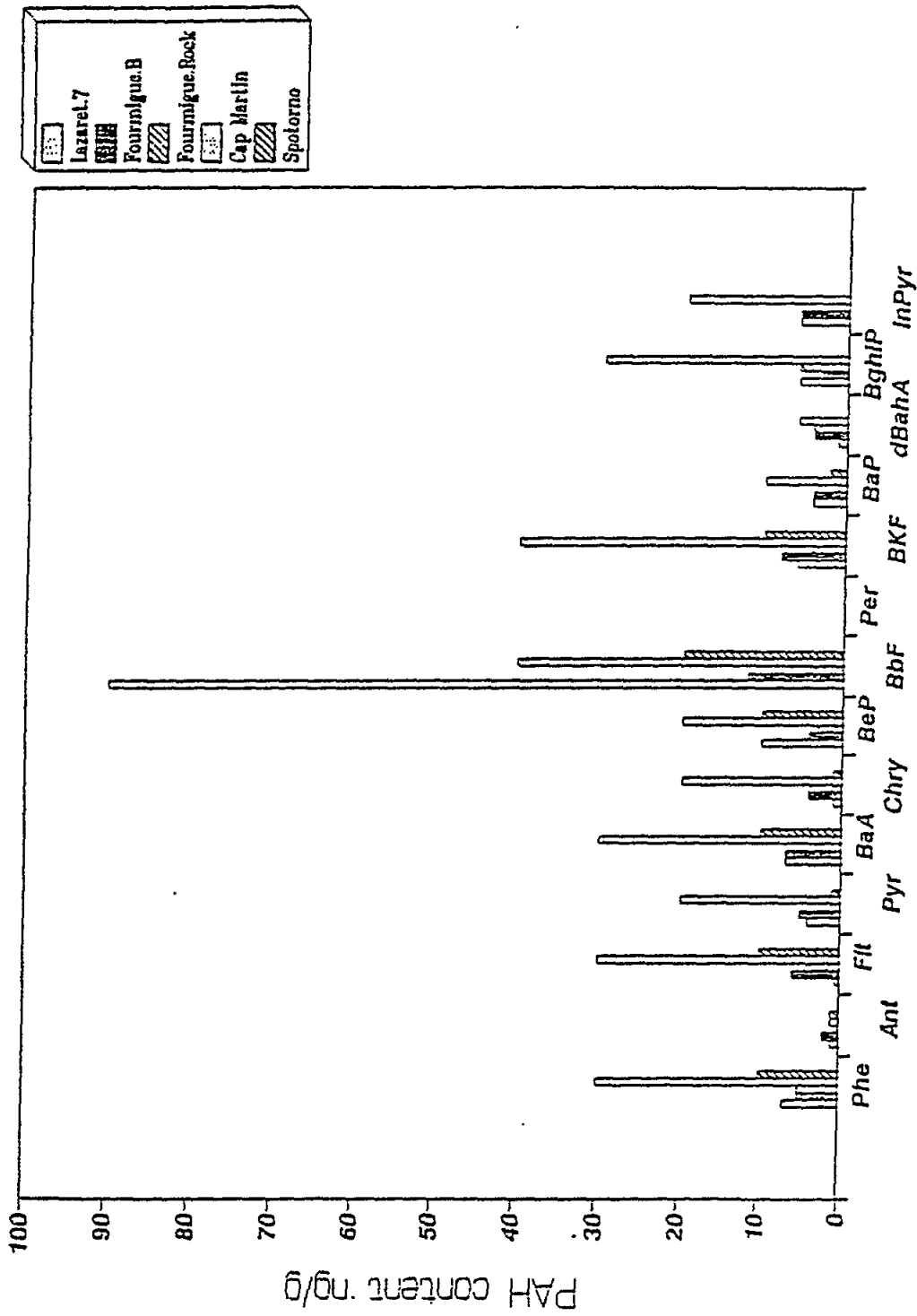
Fig. 7 Distribution des composés aromatiques dans les tissus de moules
