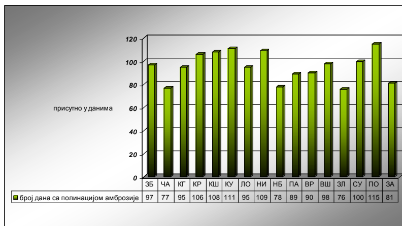
Слика 40. Укупан број дана појаве полена амброзије у години за све станице у мрежи
