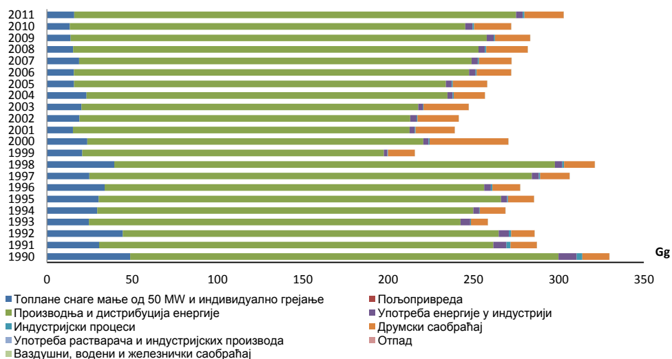
Слика 7. Емисије SO x у периоду од 1990. до 2011.године (Gg/год)
